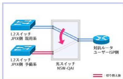
● 対抗ルータとL2スイッチの間に光スイッチ「NSW-QAI」を配置
